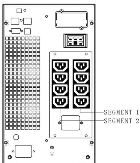
Σχήμα 11: 3KVA Tower
