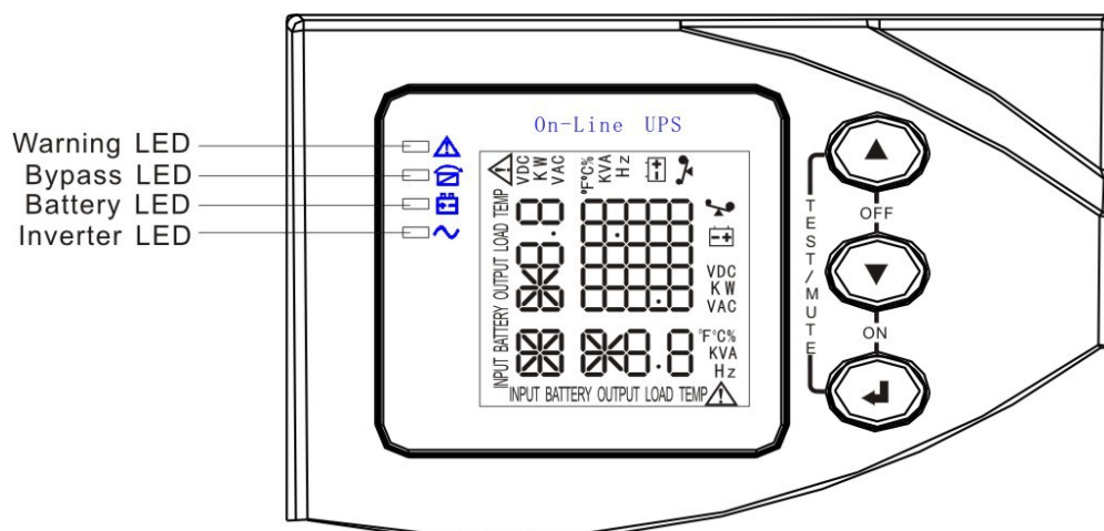
Σχήμα 3: Πίνακας ελέγχου
