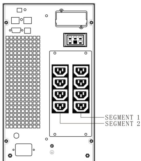
Σχήμα 10: 2KVA Tower
