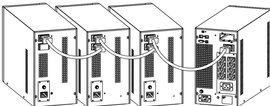
2KV/3KV Tower UPS και EBP ( S )
