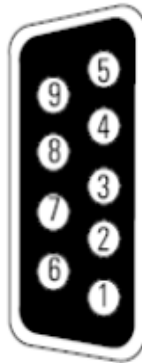
Σχήμα 5: Θύρα επικοινωνίας RS-232 (DB-9 Connector)
