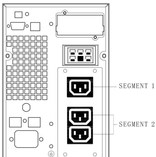
Σχήμα 9: 1KVA Tower
