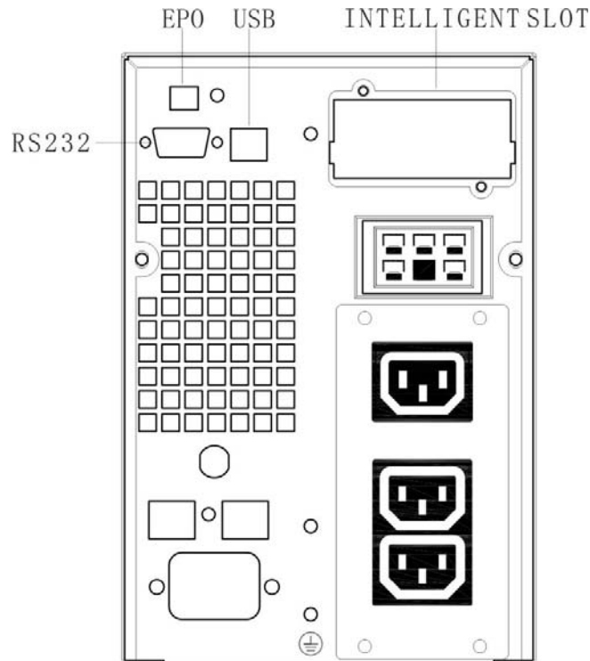
Σχήμα 4: Επιλογές επικοινωνίας και ακροδέκτες ελέγχου (1KVA μοντέλο Tower)
